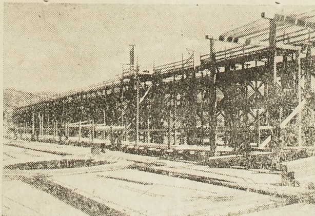
Izgradnja hale peći za proizvodnju ferolegura u Crnici
