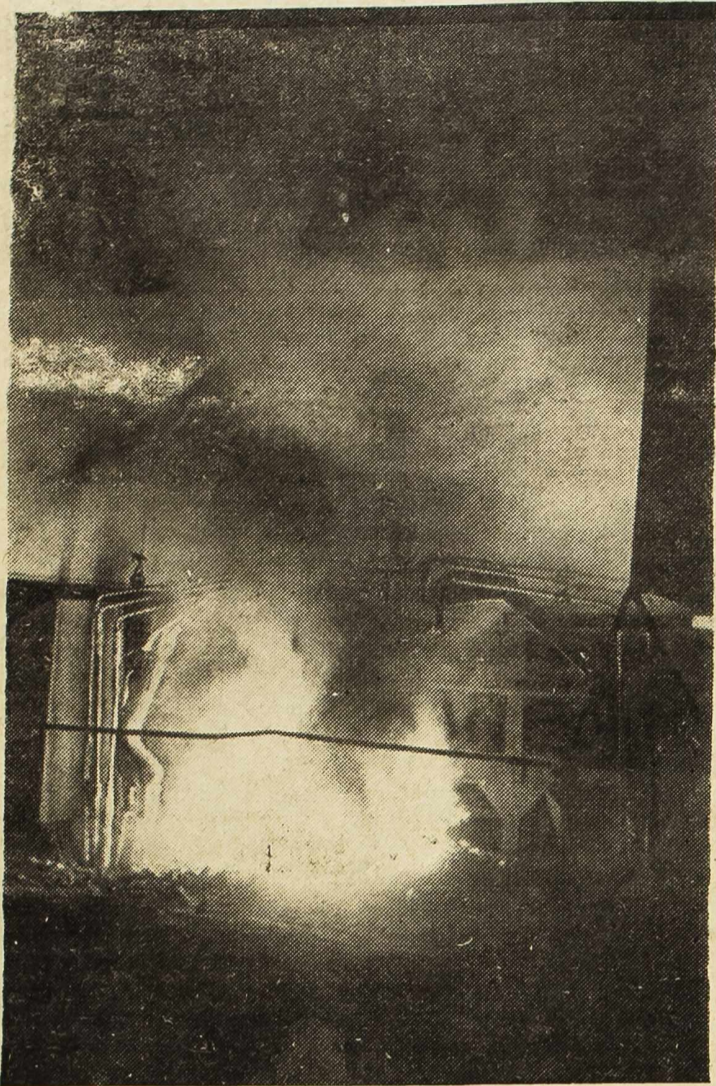
Detalj električne peći u Tvornici elektroda i ferolegura
