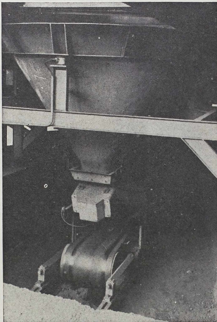
Automatska vaga za miješanje sirovina
