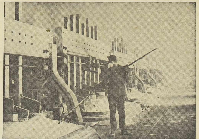
Detalj iz proizvodnog dijela Tvornice aluminija
