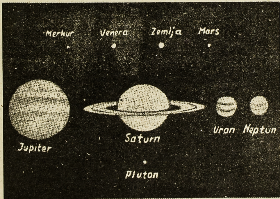
Величина планета у поређењу једних према другима
