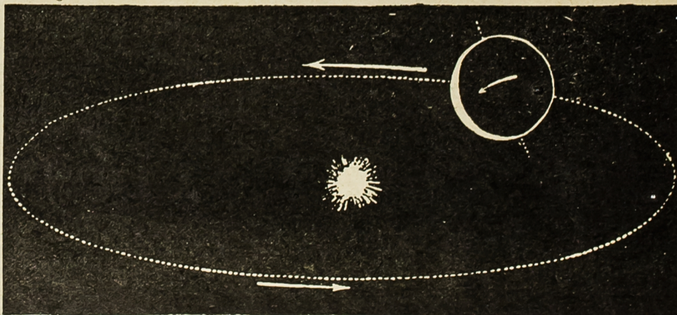
Шема кружења Земље око Сунца и њеног окретања око своје оси
